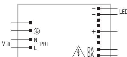
DALI diagram Collegamento DALI
